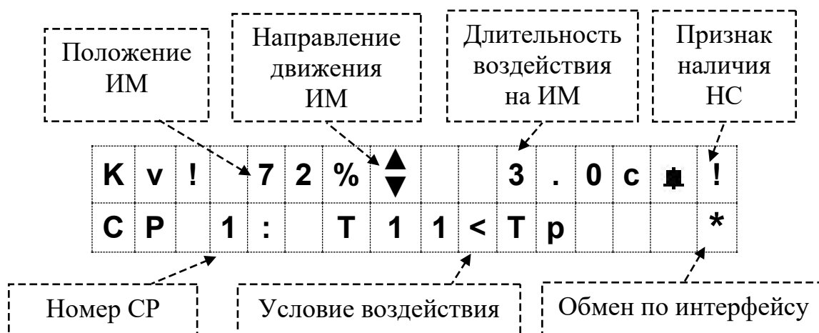
Рисунок 10 – Вид экрана индикатора в дежурном режиме
