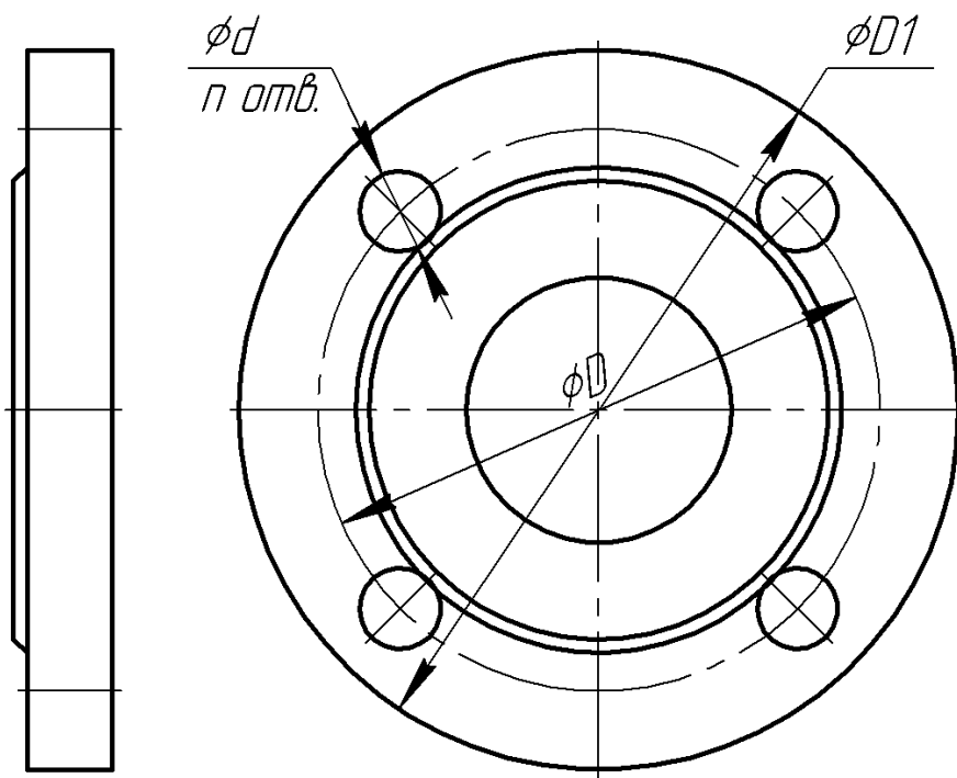
Рисунок А.2 – Присоединительные размеры фланцев
