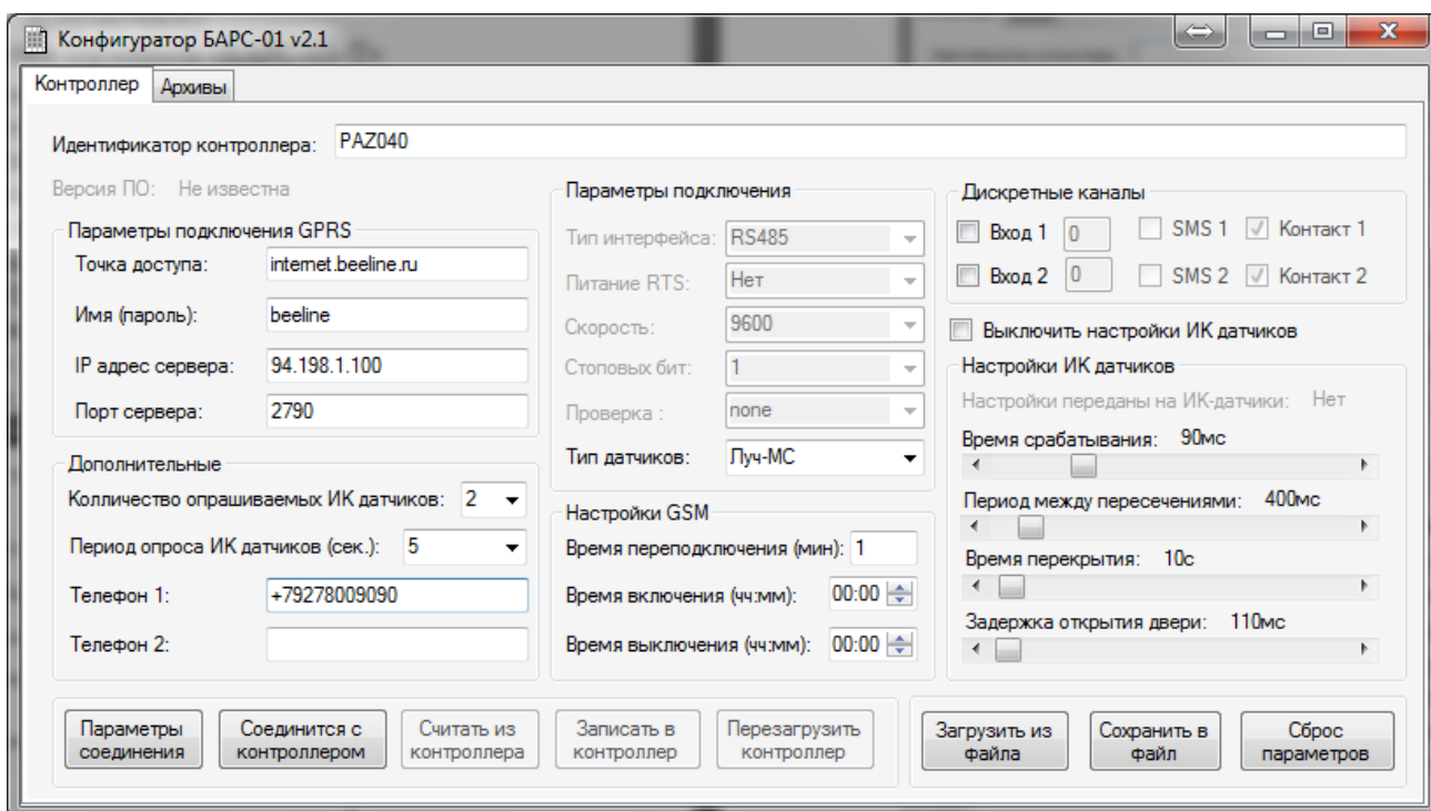
Рисунок Е.3 – Внешний вид программы настройки «БАРС-01-Т».
