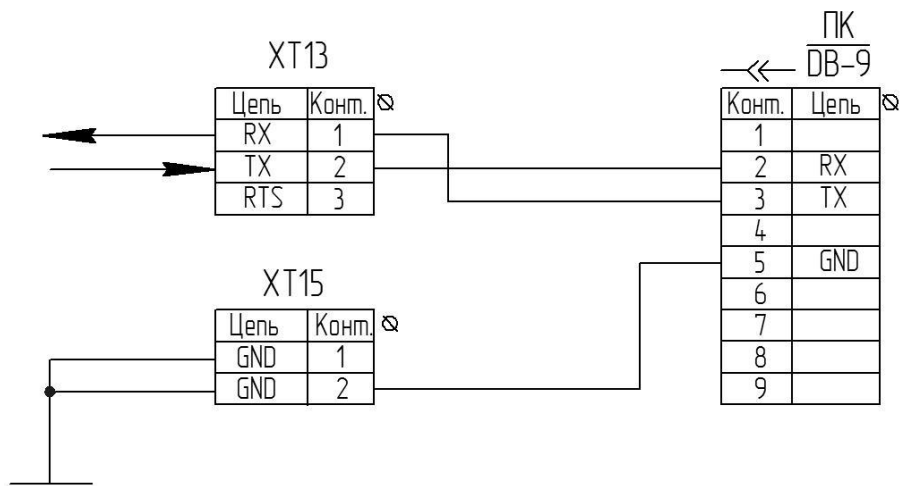
Рисунок В.3 – Схема подключения к СОМ-порту ПК.
