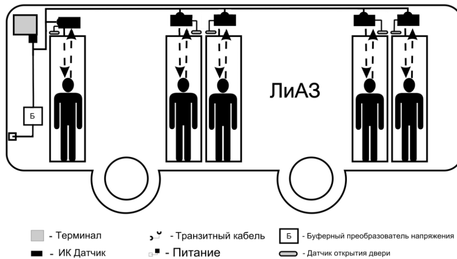
Рисунок 7 – Пример установки системы на 5-дверный автобус.
