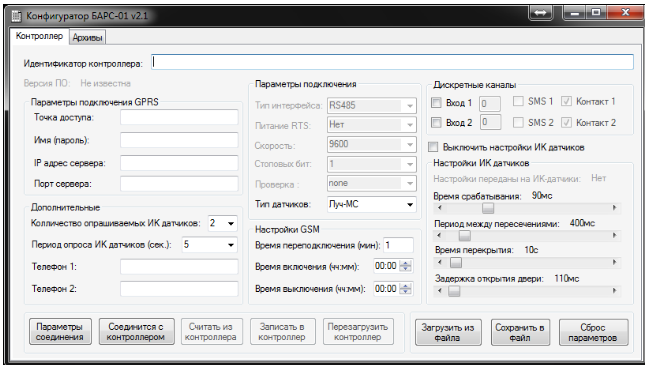
Рисунок Е.2 – Основное меню программы настройки.
