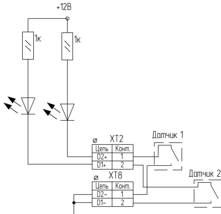
Рисунок В.4 – Схема подключения дискретных датчиков.
